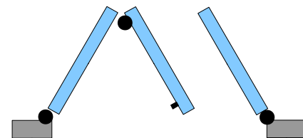
Tre ante a libro, cerniera interna apertura SPINGERE A SINISTRA Spagnoletta di chiusura su ante pieghevoli
