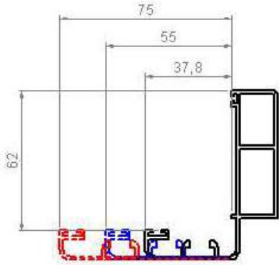
Profilo telaio con battuta 37,8/55/75 mm
