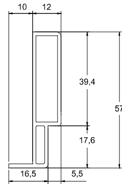
Profilo telaio con battuta 10mm
