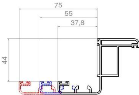
Profilo telaio con battuta 37,8/55/75 mm
