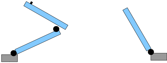
Tre ante a libro, cerniera esterna apertura SPINGERE A SINISTRA Spagnoletta di chiusura su anta pieghevoli
