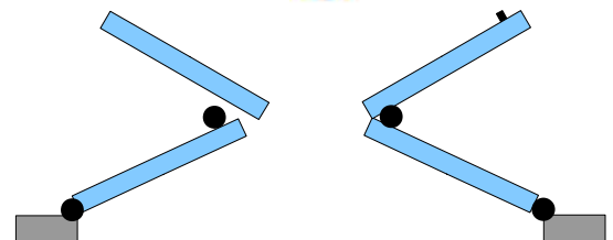
Quattro ante a libro, cerniera esterna apertura SPINGERE A DESTRA Spagnoletta di chiusura su prima anta ripieghevole DX
