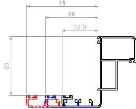
Profilo telaio con battuta 37,8/55/75 mm
